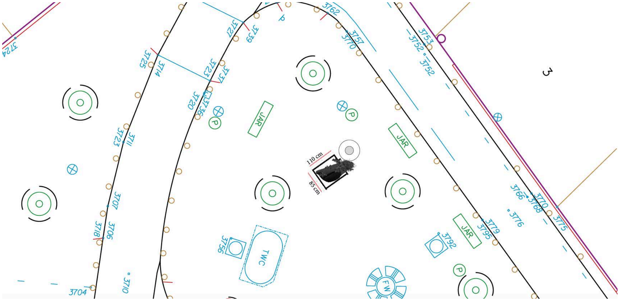
Vue en plan de la sculpture
